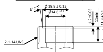
SECCIÓN PARCIAL B-B (2:1)
