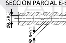
SECCIÓN PARCIAL E-E
