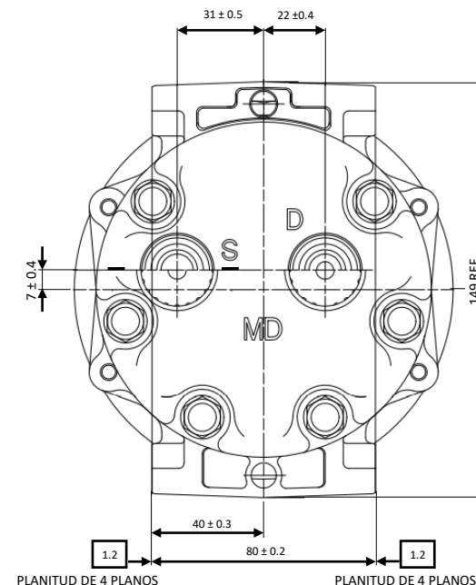
PLANITUD DE 4 PLANOS
