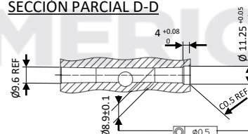
SECCIÓN PARCIAL D-D
