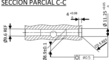
SECCIÓN PARCIAL C-C
