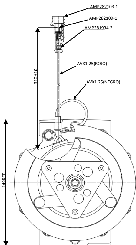
SECCIÓN PARCIAL C-C
