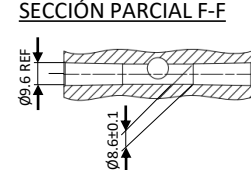
SECCIÓN PARCIAL F-F
