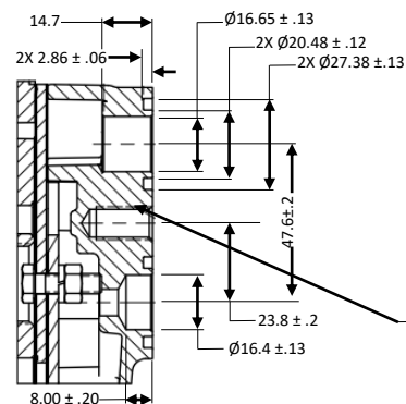
SECCION C-C ESCALA 1:1 PER QP-5109
