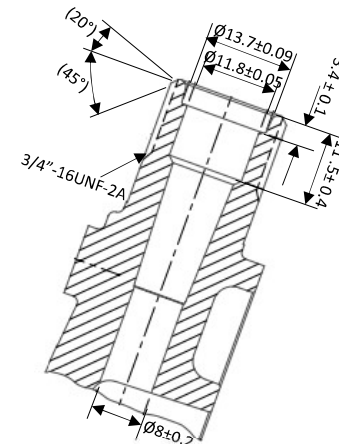
Detalle D - D
